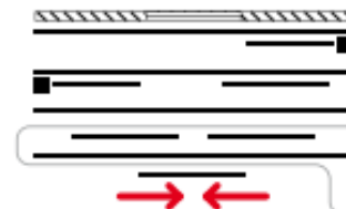
4/8 VORHANG - 6 Stoffen - Betätigungsschnur - R (f.p. hinten)
