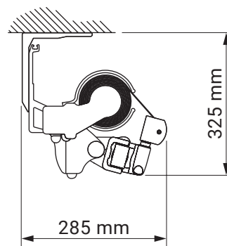
Deckenmontage
