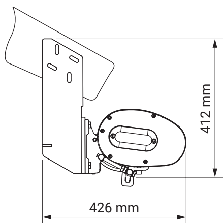
Dachsparrenmontage
