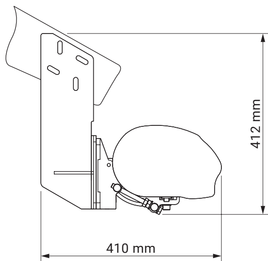
Dachsparrenmontage
