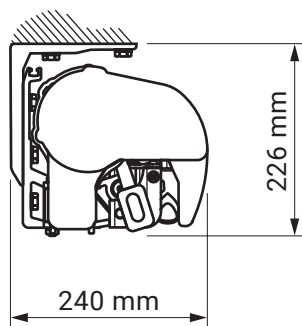
Deckenmontage
