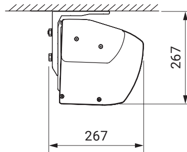
Deckenmontage
