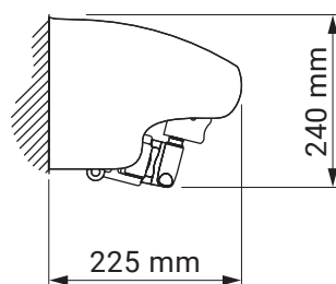
Wandmontage - Option mit Schutzdach
