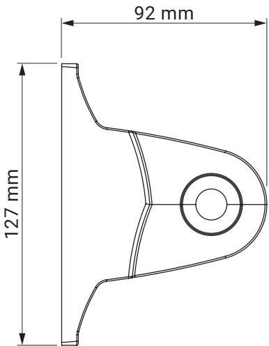
Wandhalter für Fallarm
