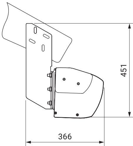
Dachsparrenmontage
