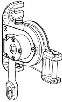
Linker Halter (Version mit Antrieb links)
