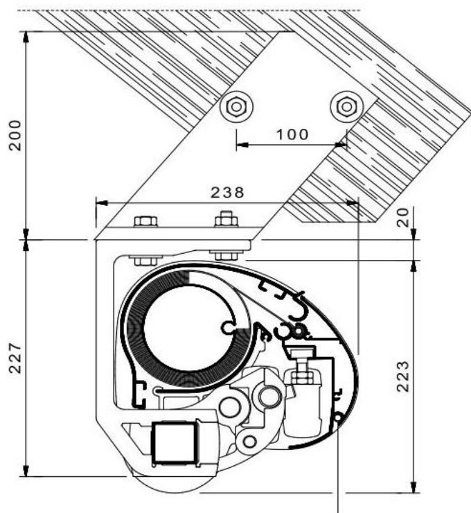
G250 Dachsparrenmontage
