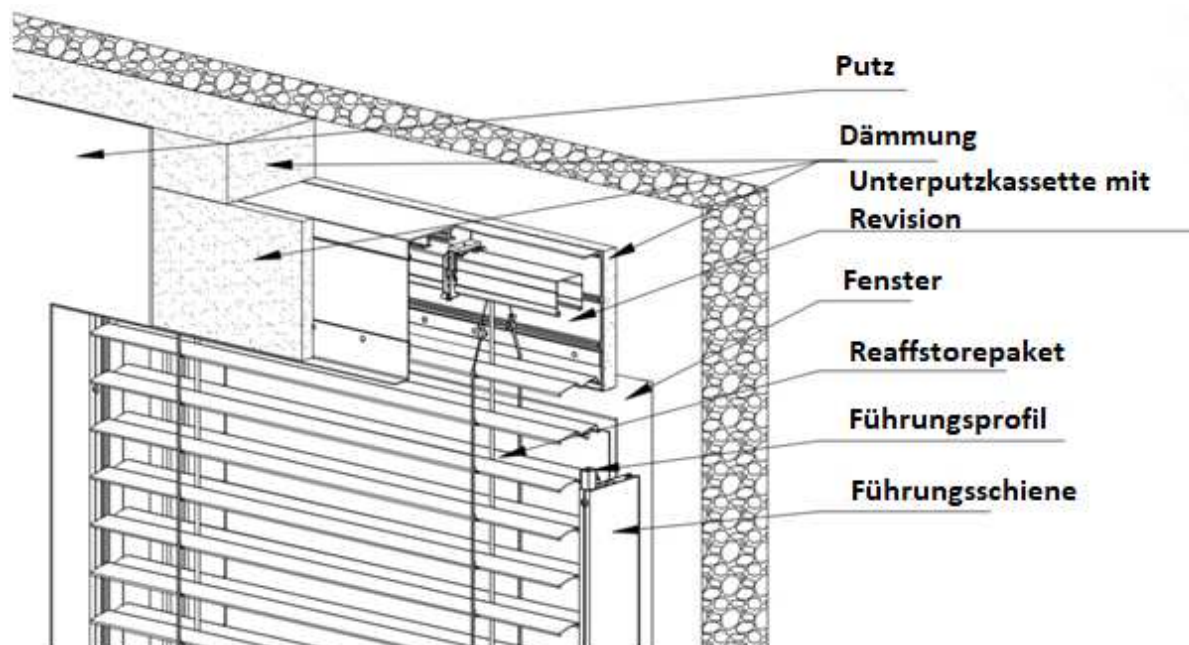
Zeichn. 10. Veranschaulichung des Raffstorensystems Z90 BOX Unterputz.
