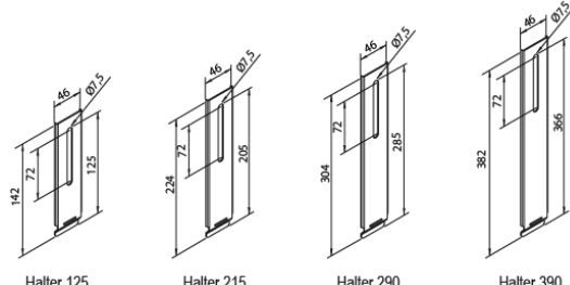
Blendenhilfshalter (4 Größen)
