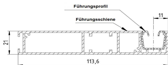
Zeichn. 9. Führungsschiene für das BOX 2 System
